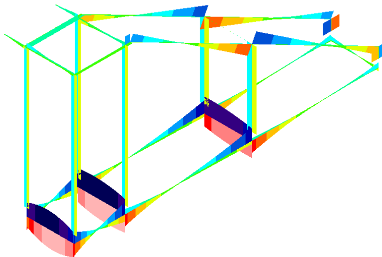
INVILUPPO TAGLIO T_x E T_y ALLO SLV
