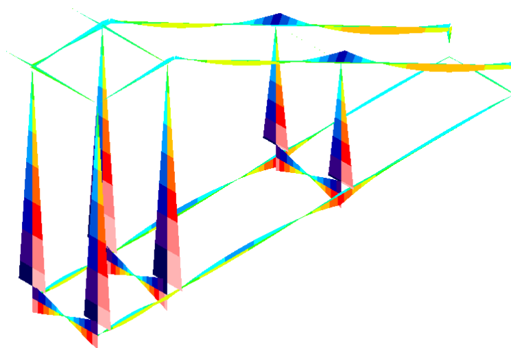
INVILUPPO MOMENTO M_x E M_y ALLO SLV
